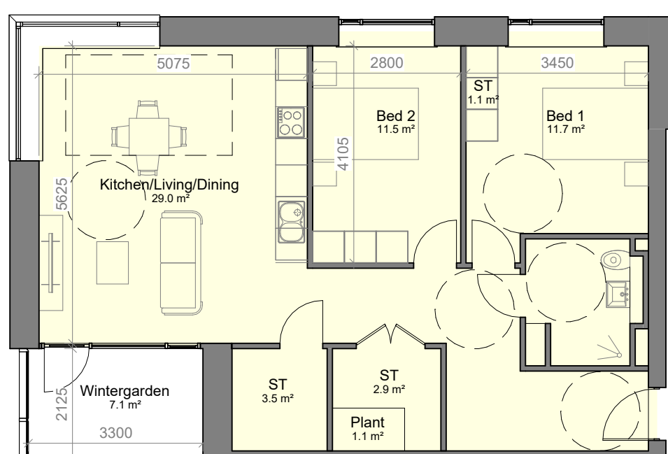
2B4P-TYPE E OD (Own Door)
