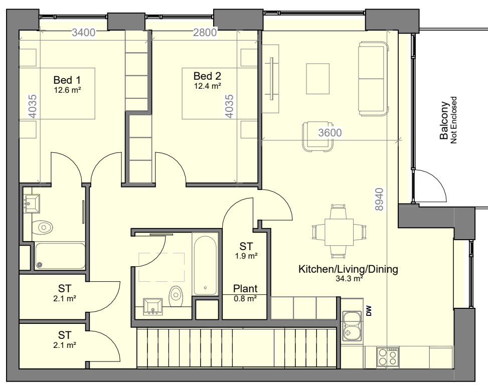
2B4P-TYPE E OD (Own Door)
